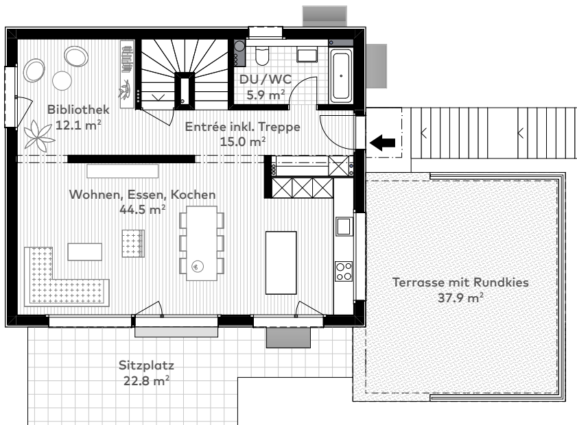
Erdgeschoss
