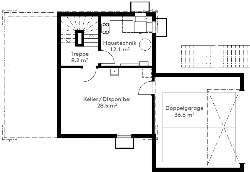
Untergeschoss
